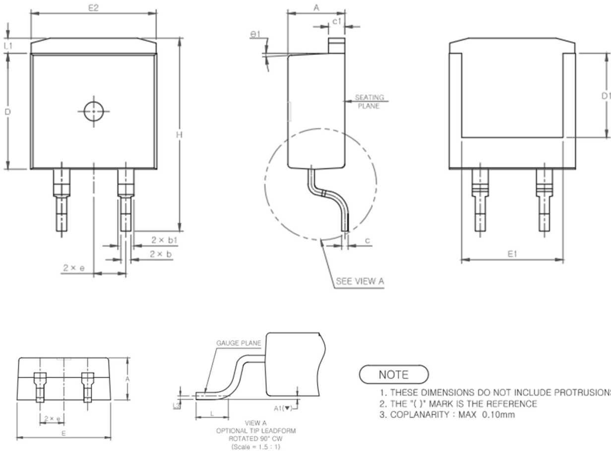
* TO-263-2L NC
